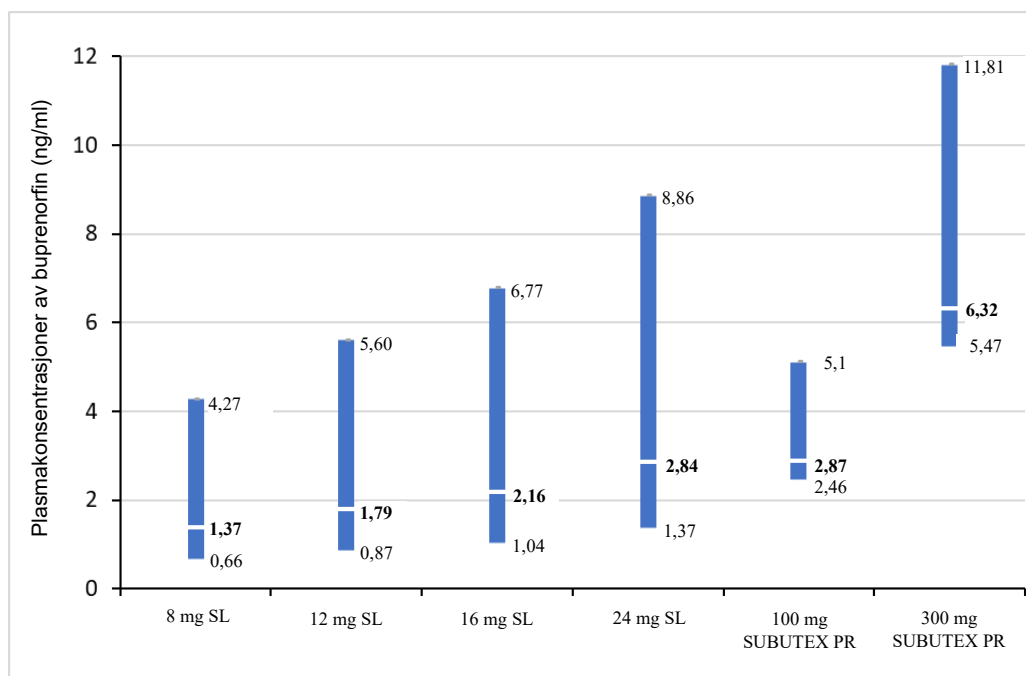
Figur 1 Sammenligning av plasmakspenning av buprenorfin ved steady-state mellom transmukosal buprenorfin og Subutex depotinjeksjonsvæske ved trough- ( C_{trough} ), gjennomsnittlig ( C_{avg} ) og maksimalt ( C_{max} ) nivå
